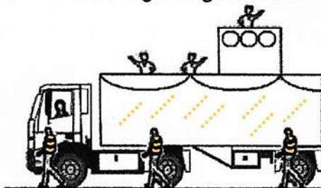
Position der Wagenengel bei Sattelzug
